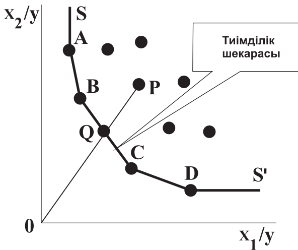
1 сурет. DEA-тәсілдің геометриялық пайымдалуы
